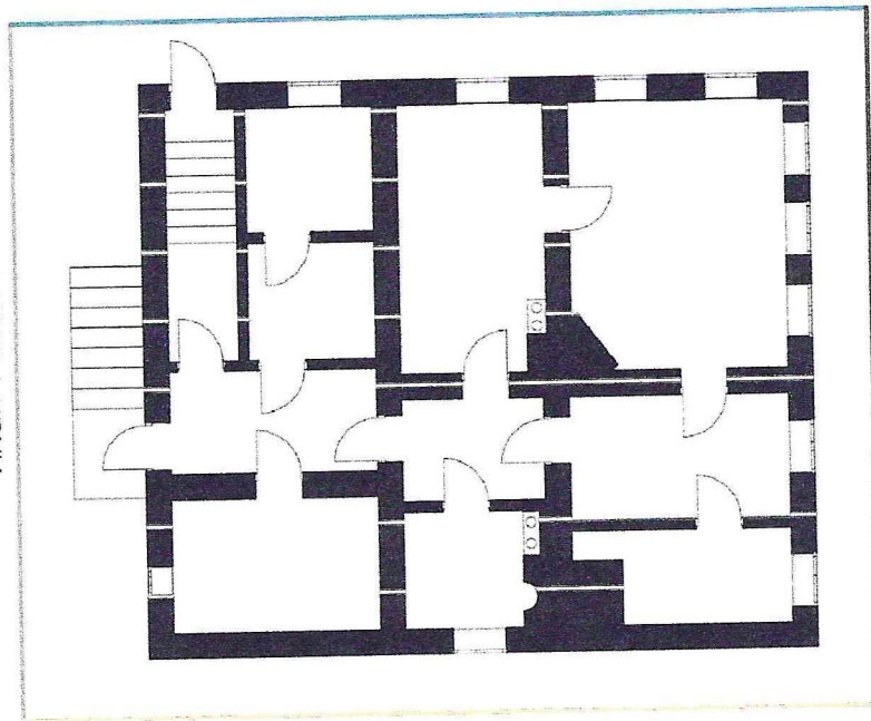
План 1 этажа
