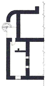
План подвала
