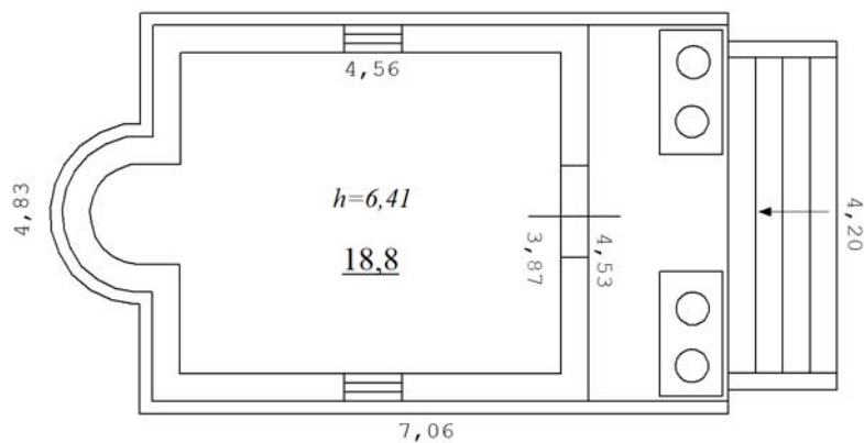
План 1-го этажа Поминальный зал
