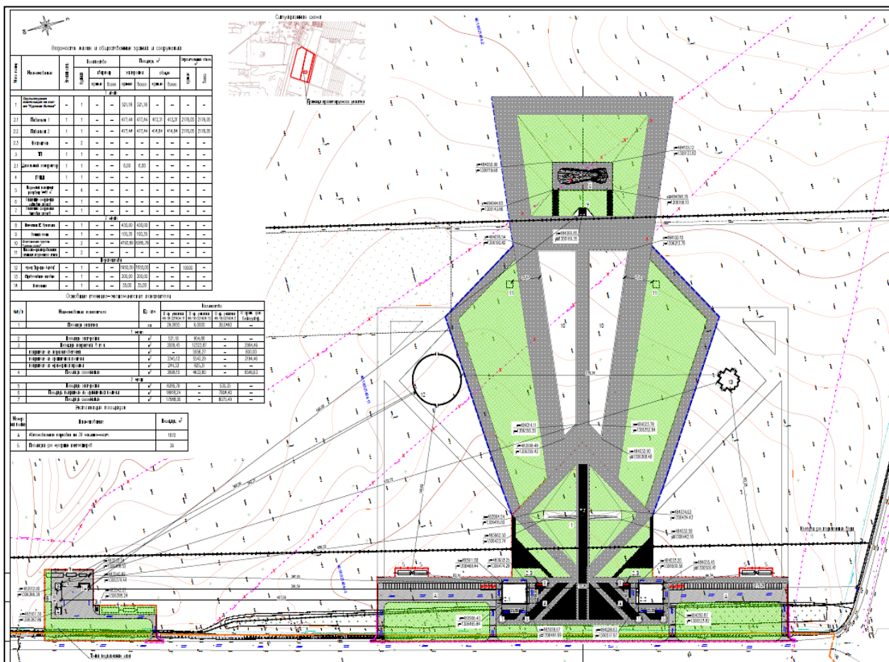
Рис. 12 | Схема планировочной организации земельного участка М 1:1000
